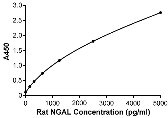
图3. Rat NGAL ELISA Kit的标准曲线。实测数据会因实验条件、检测仪器等的不同而存在差异，图中数据仅供参考。
